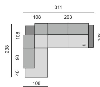
SEDACÍ SOUPRAVA: TEN40L TEN90 TEN108 TEN290P
