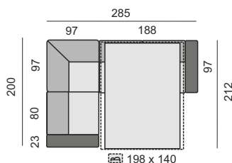
SEDACÍ SOUPRAVA: MAT23L MAT80 MAT97 MAT140PZ
