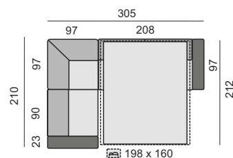
SEDACÍ SOUPRAVA: MAT23L MAT90 MAT97 MAT160PZ
